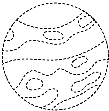
venus
